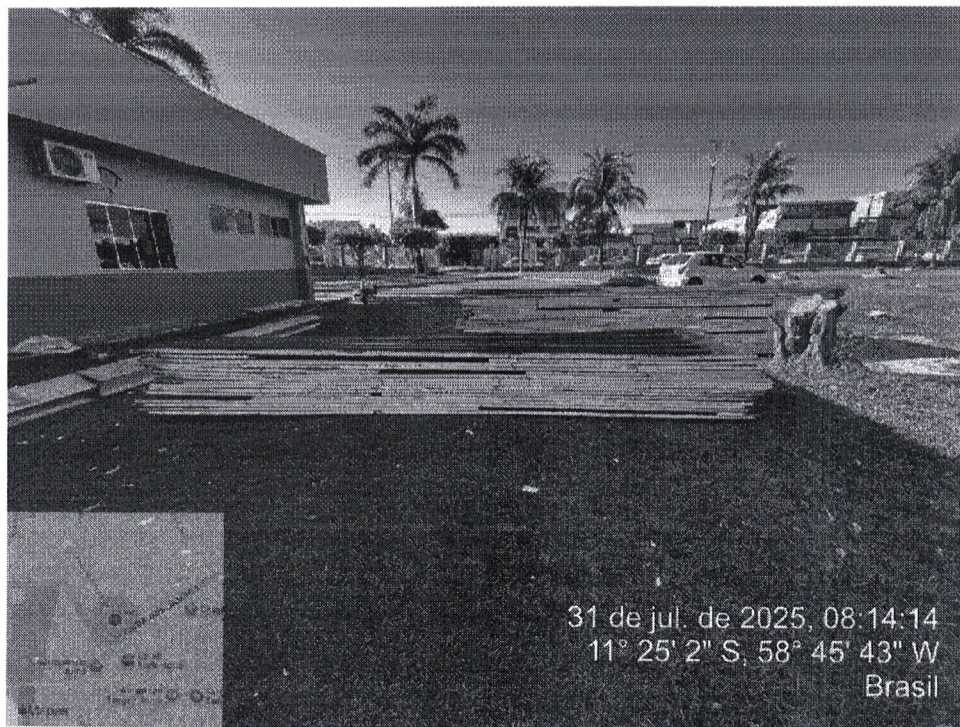
Foto 19 – remoção de telhas, calhas, chapim e rufos, itens 2.1.1 e 2.1.3 Fonte: Prefeitura Municipal de Juína
