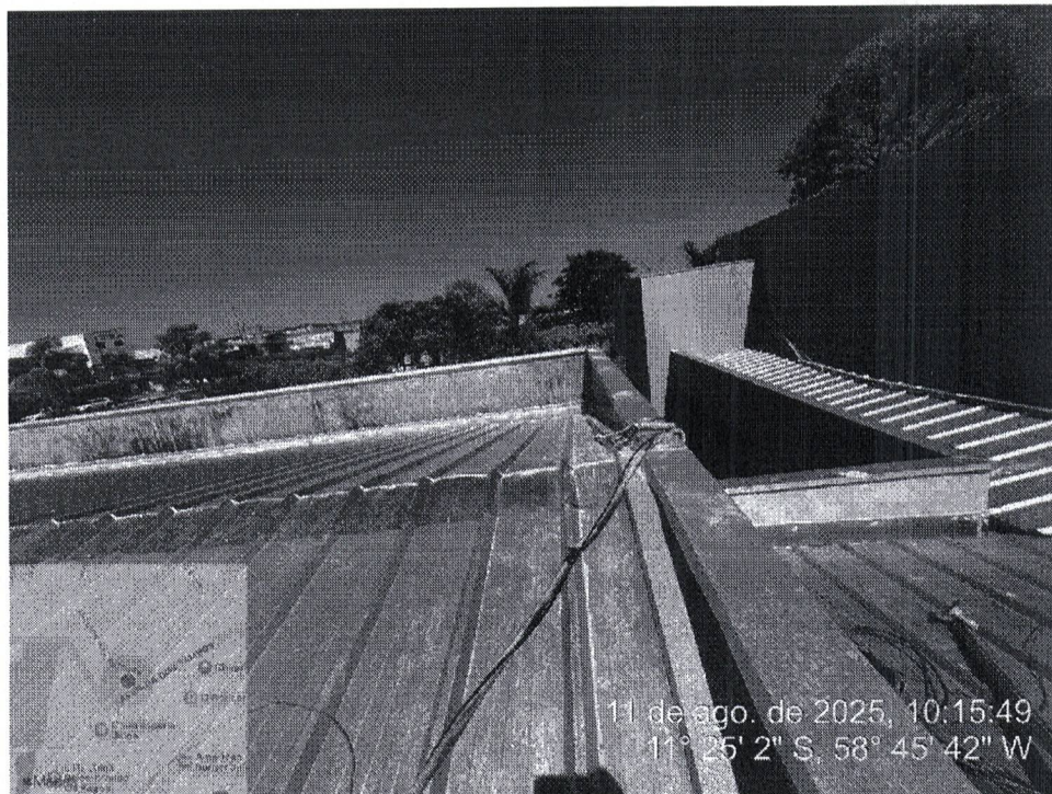
Foto 23 – Troca de telhamento, calhas, chapim e rufo, itens 2.1.2, 2.1.4, 2.1.5 e 2.1.6 Fonte: Prefeitura Municipal de Juína
