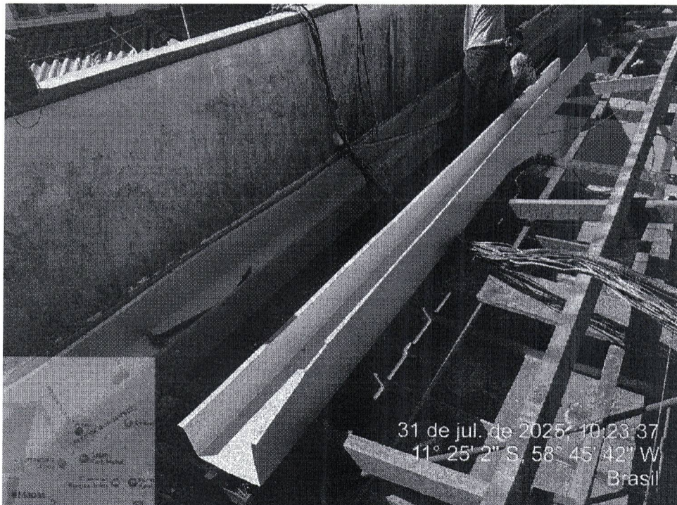
Foto 26 – Troca de telhamento, calhas, chapim e rufo, itens 2.1.2, 2.1.4, 2.1.5 e 2.1.6 Fonte: Prefeitura Municipal de Juína
